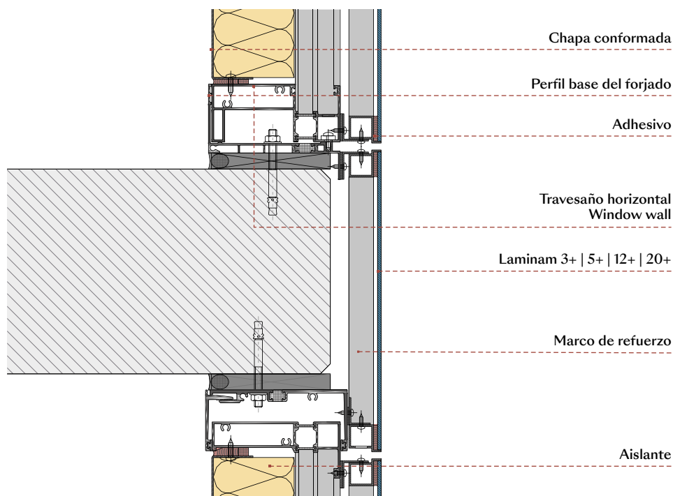
Ejemplo de una losa anclada con un sistema estructural enrasado con el exterior
